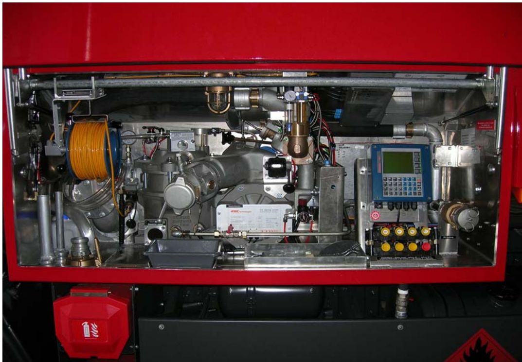
Abgabeeinrichtung in Integriertem App. Schrank auf der rechten Fahrzeugseite
