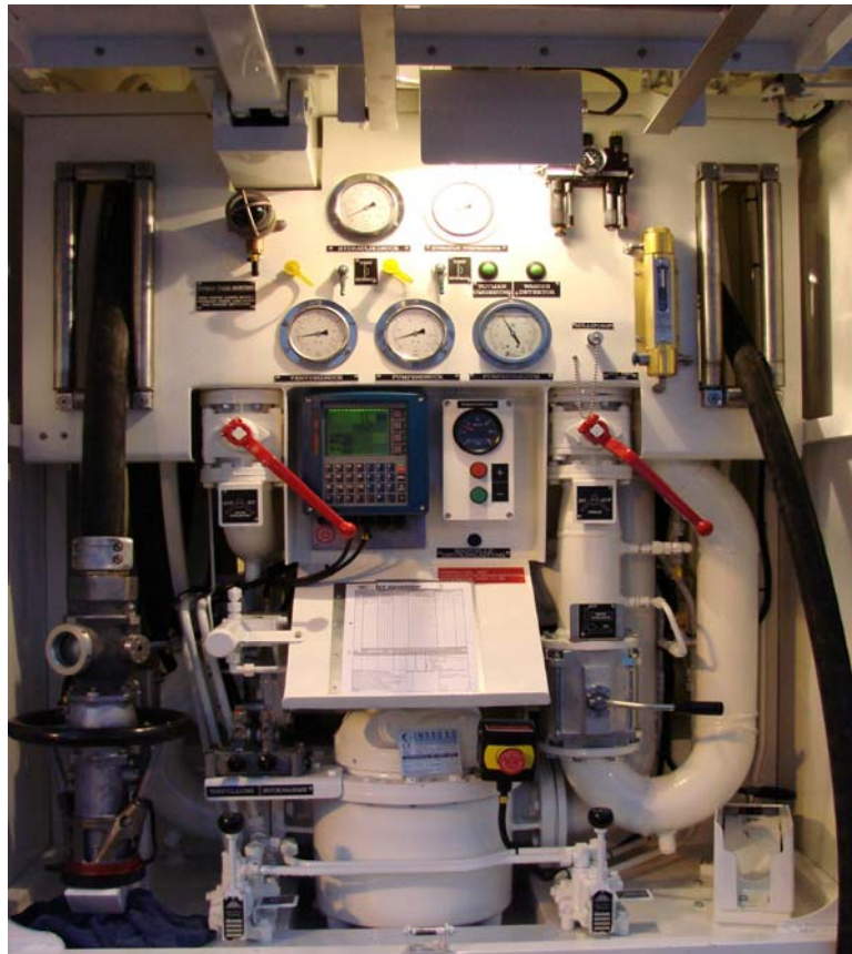
Abgabesystem mit Gormann Rupp Mediumpumpe, Haar Inline Druckregelung, Smith Meter und Bartec TMU
